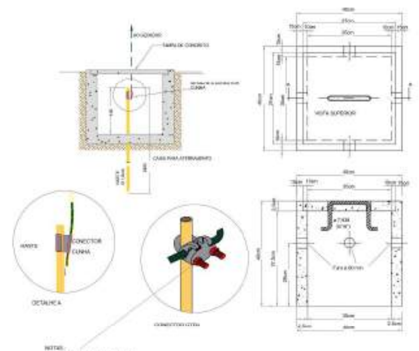
DETALHAMENTO DO ATERRAMENTO
