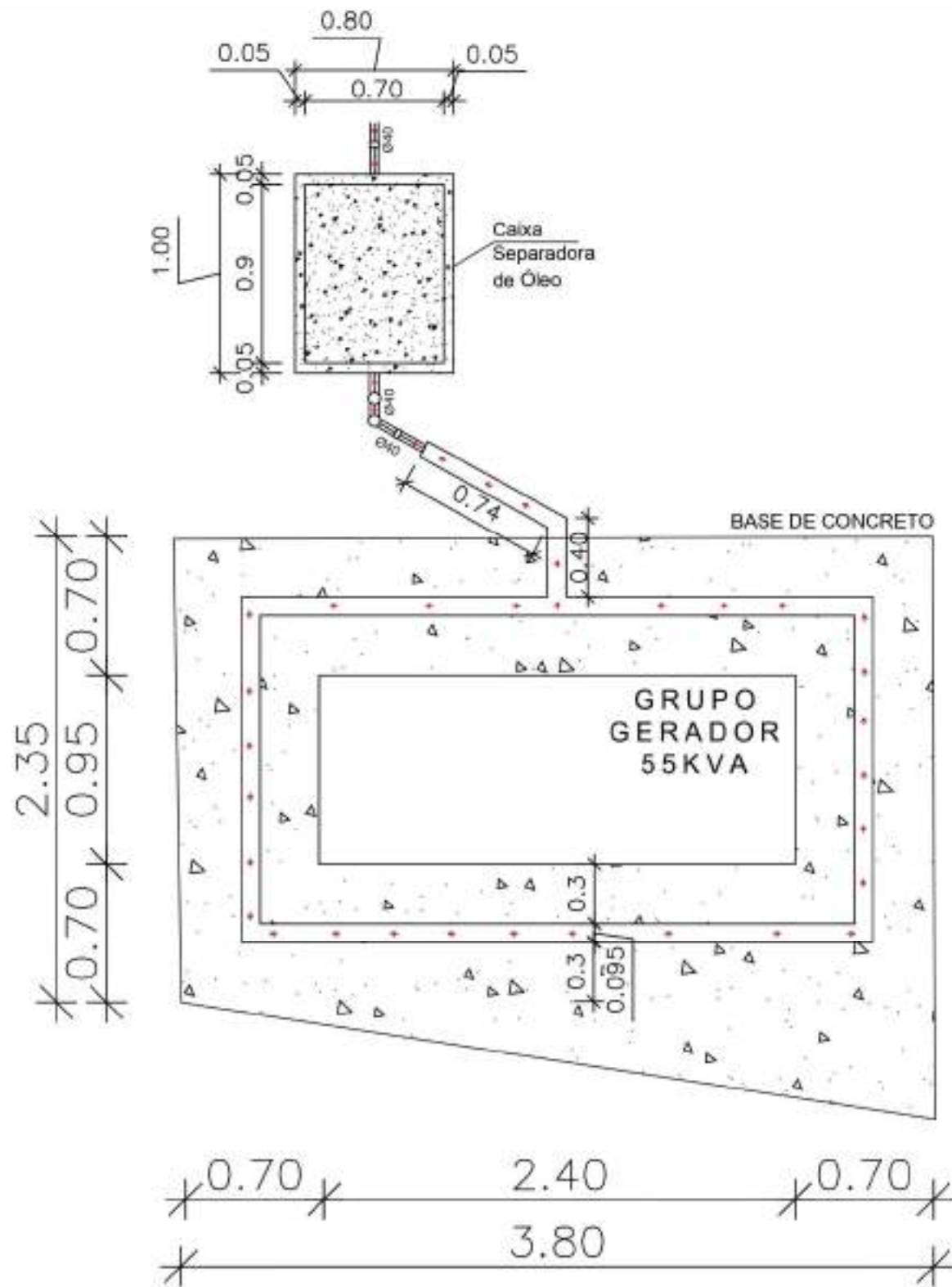
DRENAGEM OLEOSA – ESC. 1/100
